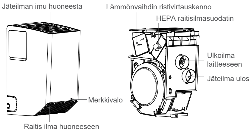
Rakenneselostus kaaviona
